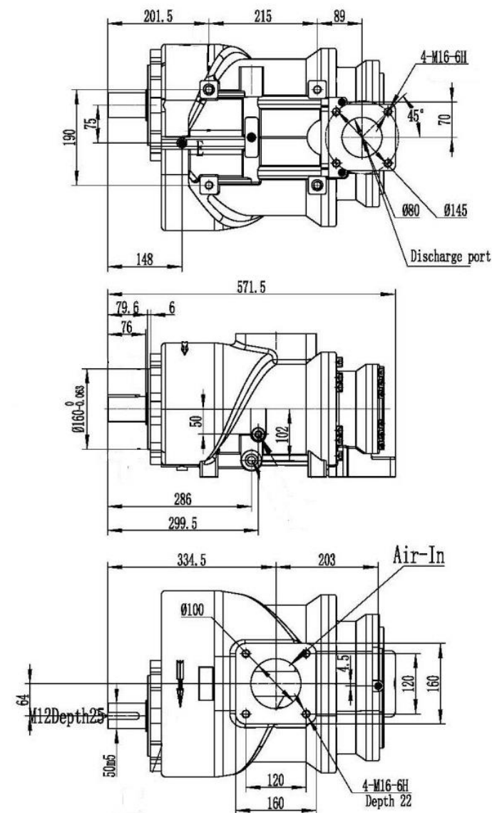
Рисунок 4. Винтовой блок YNE163RA.
