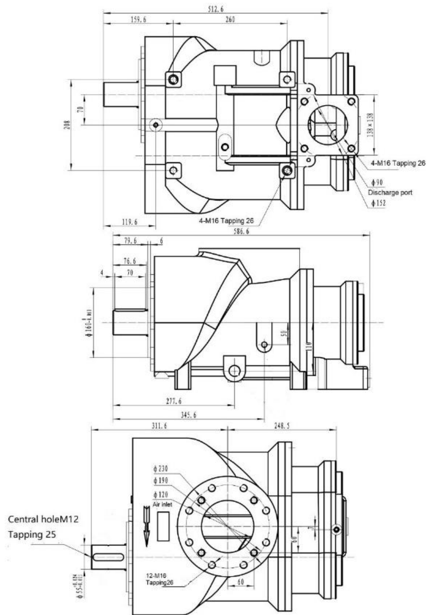
Рисунок 3. Винтовой блок YNE178RA.
